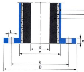
Rohr/Rohrbogen mit Festflansch
