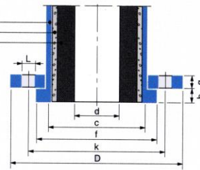
Rohr/Rohrbogen mit festem Bund und losem Flansch
